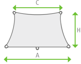
TRAPEZOIDI SEINÄKIINNITYKSEEN
